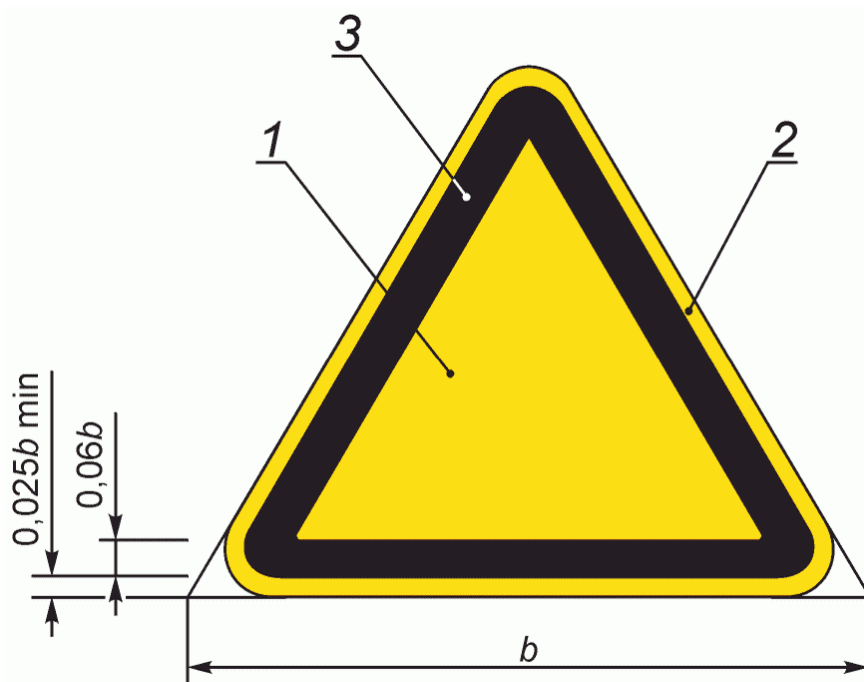
b - сторона треугольника; 1 - основная поверхность; 2 - кант; 3 - кайма
