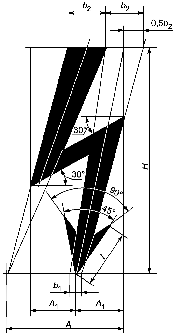
Рисунок Н.1 - Графический символ электрического напряжения
