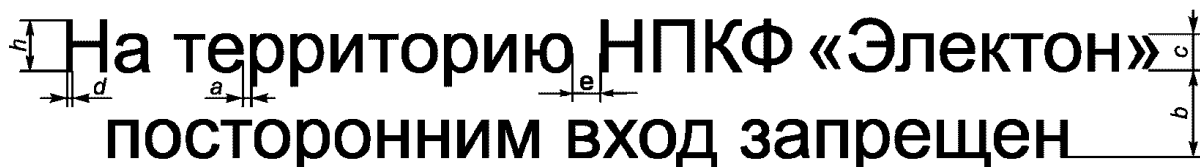
Рисунок Р.1 - Пример выполнения поясняющей надписи
