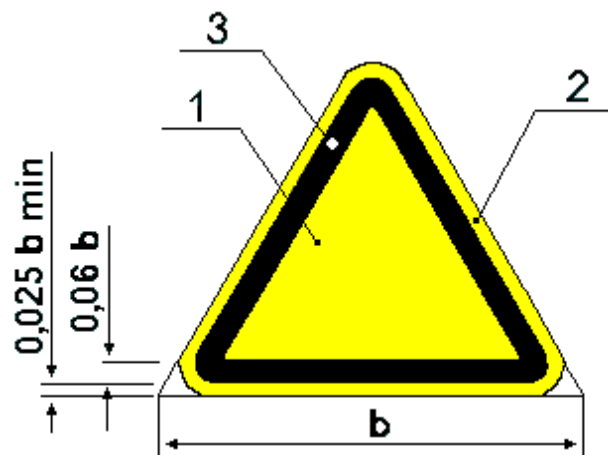
b – сторона треугольника; 1 – основная поверхность; 2 – кант; 3 – кайма Рисунок 2 – Основа цветографического изображения и соотношение размеров предупреждающих знаков безопасности
