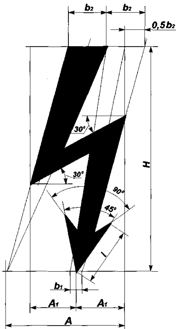
Рисунок Л.1 — Графический символ электрического напряжения
