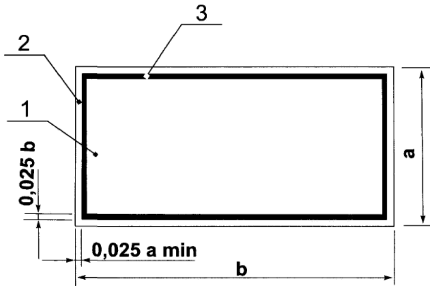
a, b – стороны прямоугольника ( 2a = b ); 1 – основная поверхность; 2 – кант; 3 – кайма Рисунок 7 – Основа цветографического изображения и соотношение размеров дополнительных знаков безопасности
