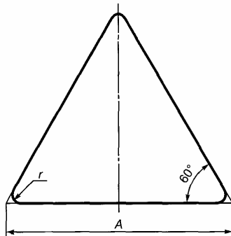
Рисунок Д.1 - Размеры треугольных знаков
