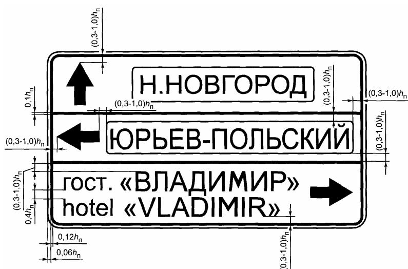
Рисунок Г.4 - Пример компоновки знака индивидуального проектирования 6.10.1
