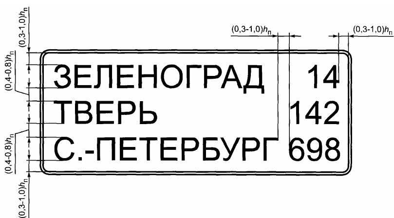
Рисунок Г.5 - Пример компоновки знака индивидуального проектирования 6.12
