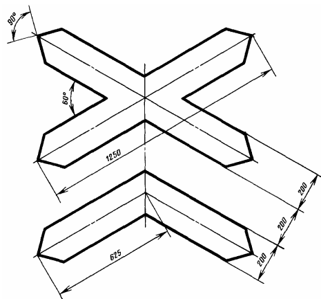
Рисунок Д.2 - Размеры знаков 1.3.1, 1.3.2
