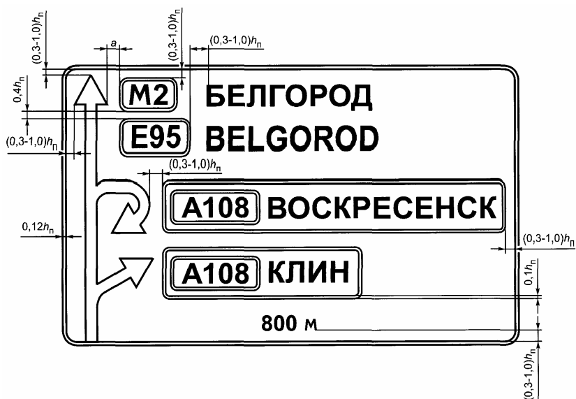
Рисунок Г.3 - Пример компоновки знака индивидуального проектирования 6.9.1
